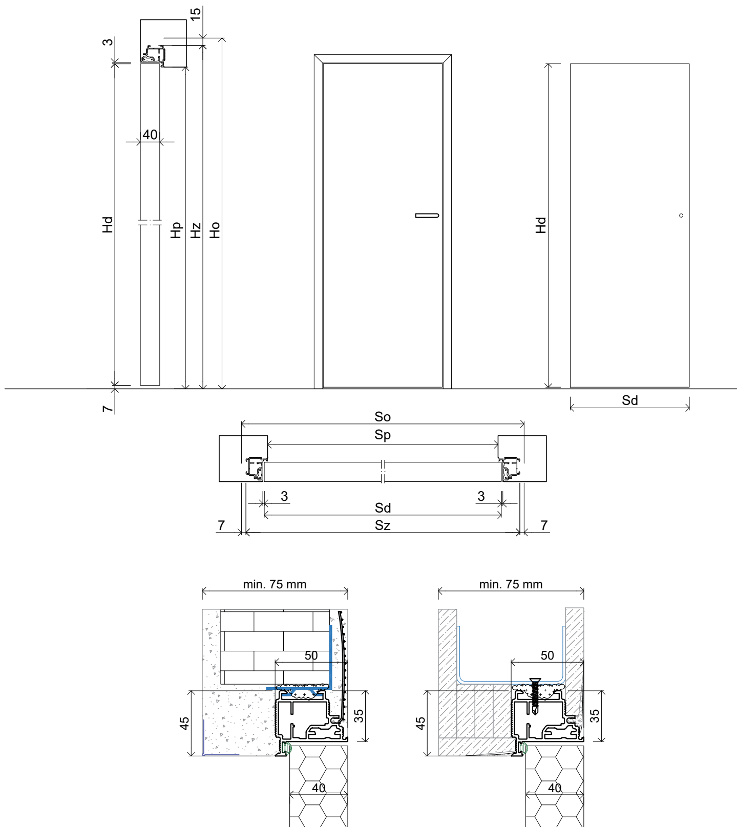
Wymiary standardowe dla drzwi otwieranych na zewnątrz
